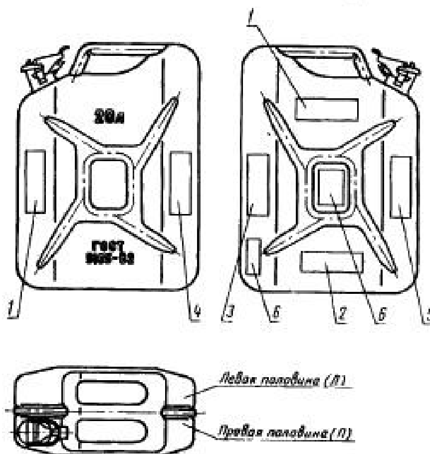
Схема вырезки пластины для испытаний
