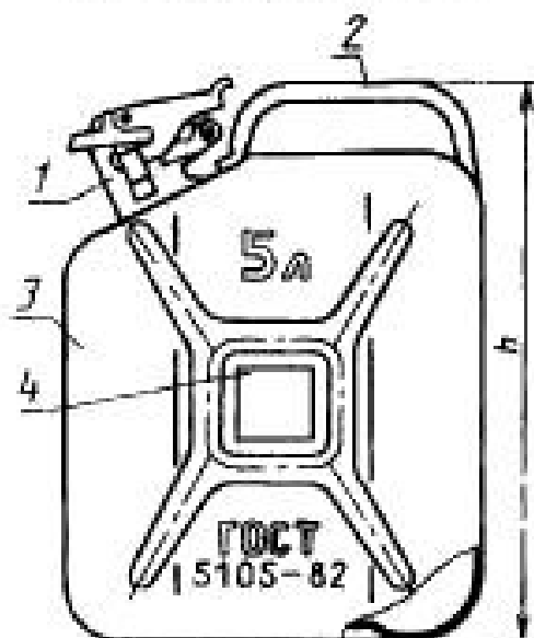
Канистра вместимостью 5 дм 3
